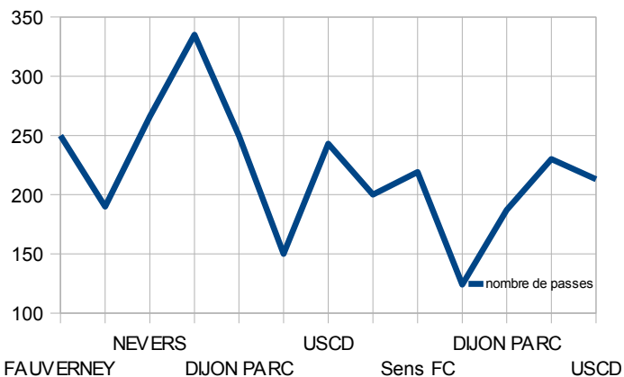
Nombre de passes par match
