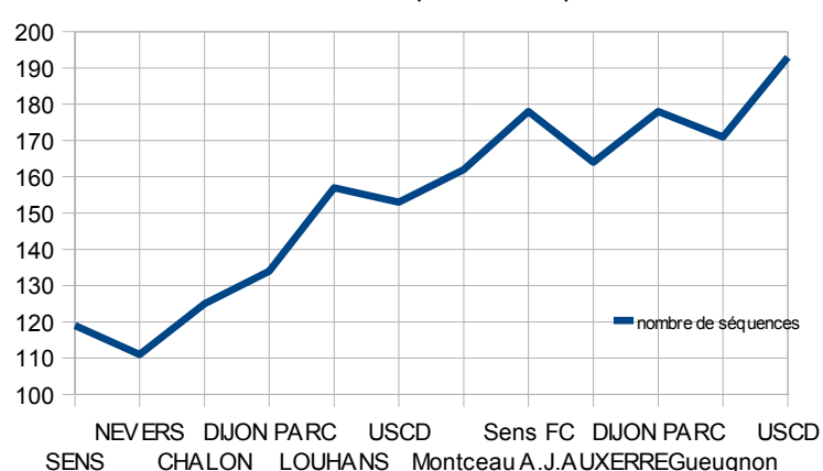
Nombres de séquences de passes
